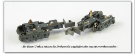
KT-101.6: Einbau Rapido-Kupplung an zwei Drehgestelle der Kato BEX-Panoramawagen, inkl. Material, ohne Drehgest.
