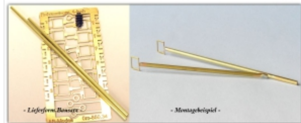
0m-850.32: Rohrausleger mit Fahrleitungshalter, für 4mm-H-Profil, Bausatz, 1 Stück
