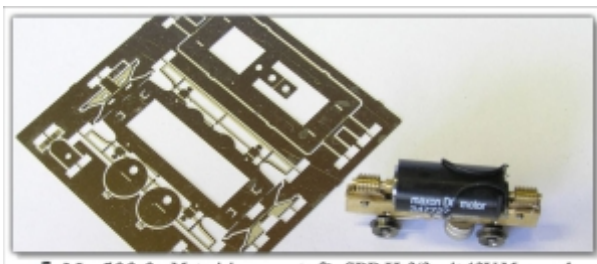
Ne-500.0: Motorisierungssatz für SPB He2/2 mit 12V-Maxon-Antrieb fertig vormontiert und Rahmenätzteil (Bausatz)
